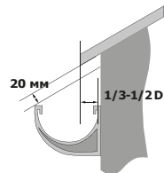
Рис. 1: Определение положения желоба относительно кровельного свеса
